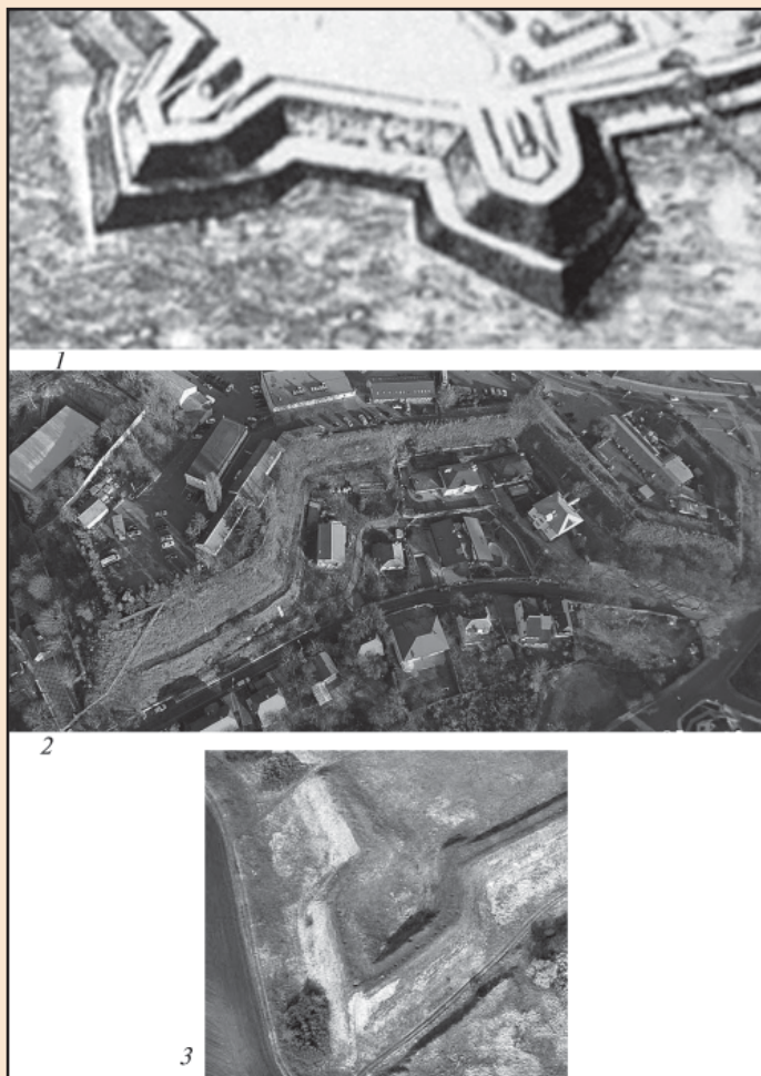
Іл. 7. Bastiони Печерської фортеці початку XVIII ст. за реконструкцією О.В. Сіткарьової (1) та сучасним фото (2); bastiон Іванівського форту в Харківській обл. (3)
