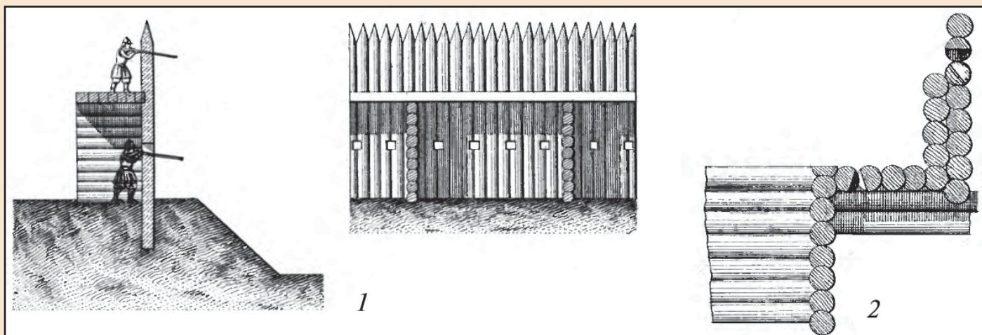
Іл. 4. Можливий вигляд однорядного острогу (1) та обламів (2) Старокиївської фортеці (за Ф.Ф. Ласковським)
