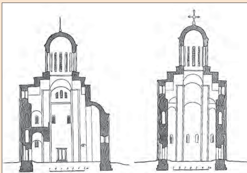
Продольні й поперечні зрізи П'ятницької церкви (реконструкція). За М. Холостенком
