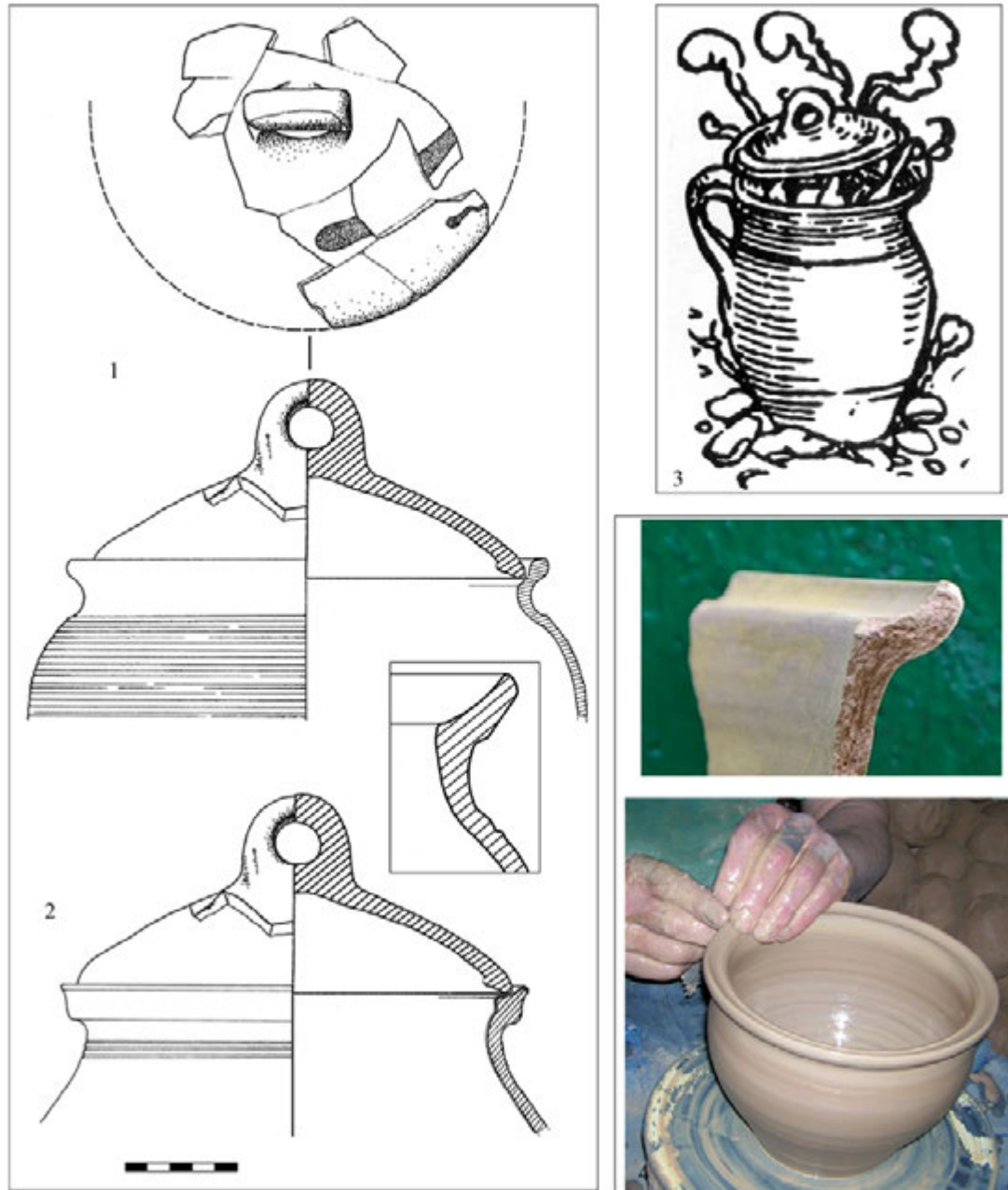
Іл. 5. Покришка I типу і варіанти її припасування до різних вінець горщиків (1, 2), зображення в стародруках XVI ст. (3) (за: Gardawski, Kruppe 1955, tabl. 36), виготовлення вінець з виїмкою під покришку сучасним гончарем (4)
