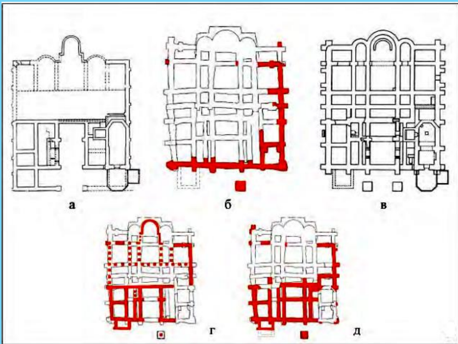
Іл. 3. Порівняння креслень плану Десятинної церкви К. Лохвицького (а) та М. Єфимова (в) із планом, створеним під час розкопок 2005–2011 років (б); збережені частини фундаментів, зафіксовані К. Лохвицьким (г) та М. Єфимовим (д)
